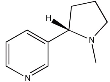
Nicotine
