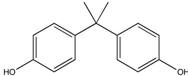
Bisphenol A
