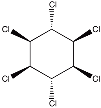
Lindane
