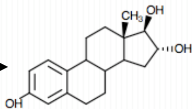
Estriol
