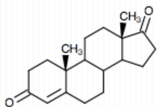
Androstenedione
