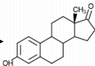
Estrone
