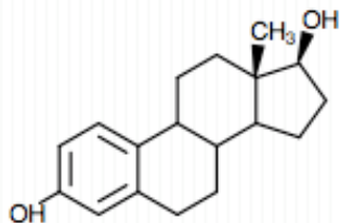
Estradiol
