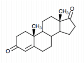
Androstenedione
